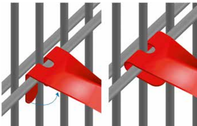
Stabile Querstreben verhindern Verformungen
